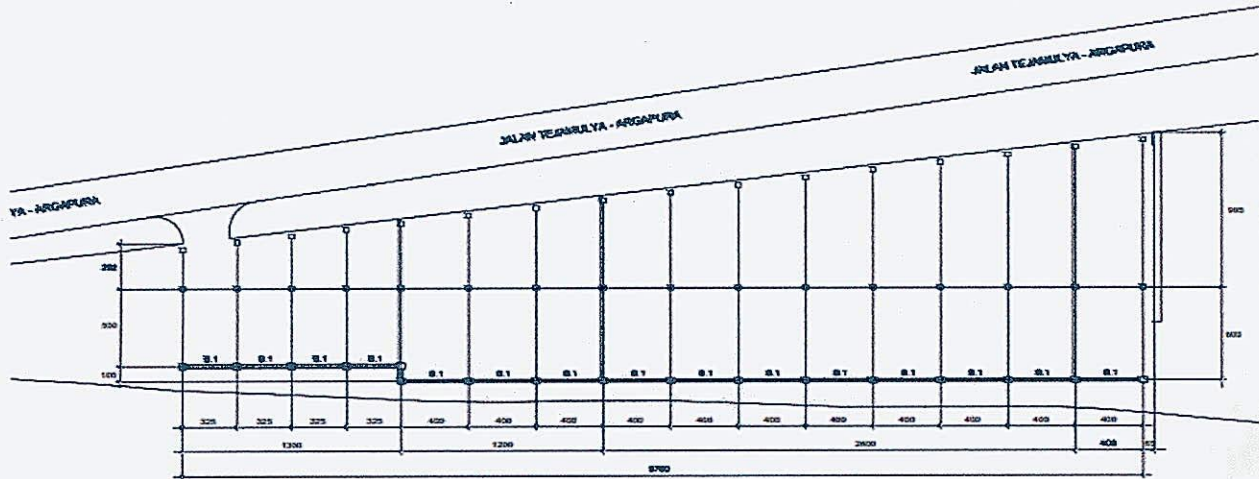
DENAH PENEMPATAN B.1 20/40 Cm
